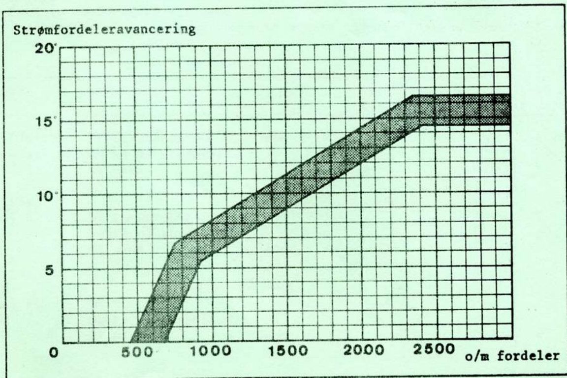
Avanceringskurve DS2o-ID2o
