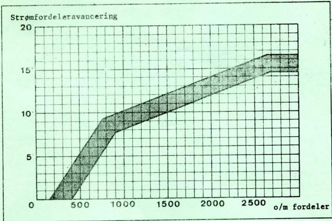
Avanceringskurve DS2o-ID2o
